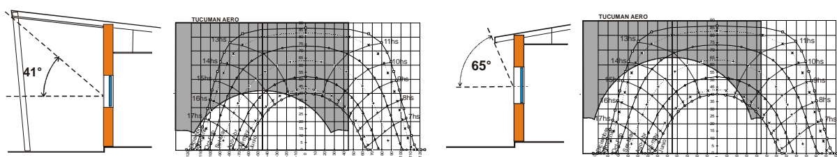
Figura 8: Determinación del período de obstrucción sobre muros considerando galería y alero.
